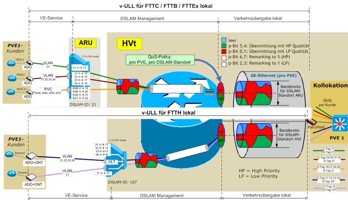
Abbildung 14: v-ULL 2.0 lokal Service- u. Netzarchitektur FTTC/FTTB/FTTH sowie FTTEX (VLANs sowie Bandbreiten sind exemplarisch)
