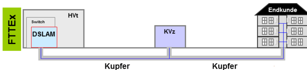
Abbildung 4: FTTEx Allgemein
