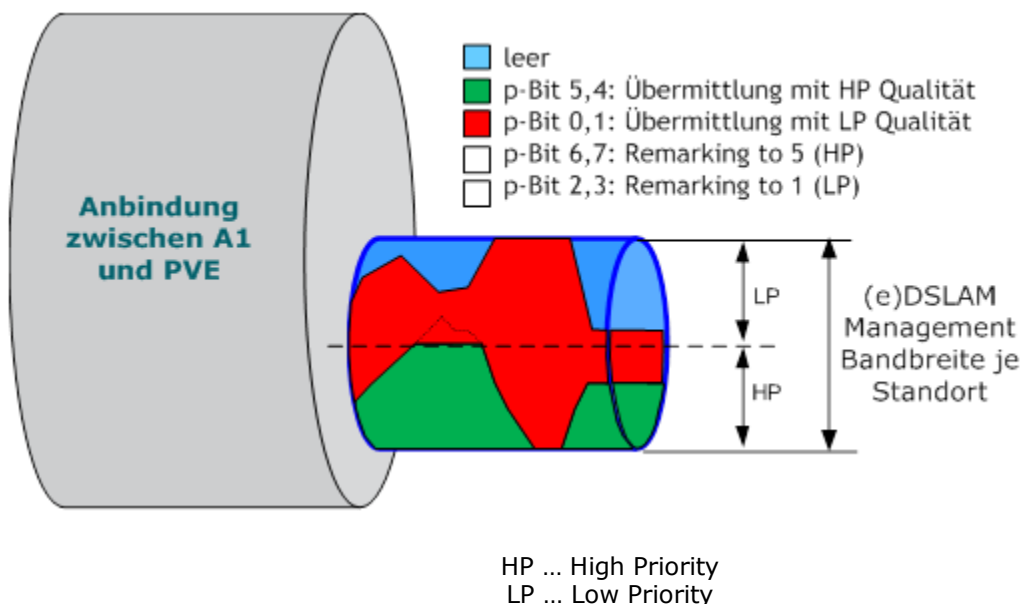
Abbildung 15: Verhalten der Daten-Frames entsprechend dem p-Bit-Marking des S-Tag
