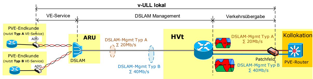
Abbildung 11: DSLAM Management lokal je Standort mit dem A-DSLAM Management A und dem B-DSLAM Management mit zwei getrennten Verkehrsübergaben
