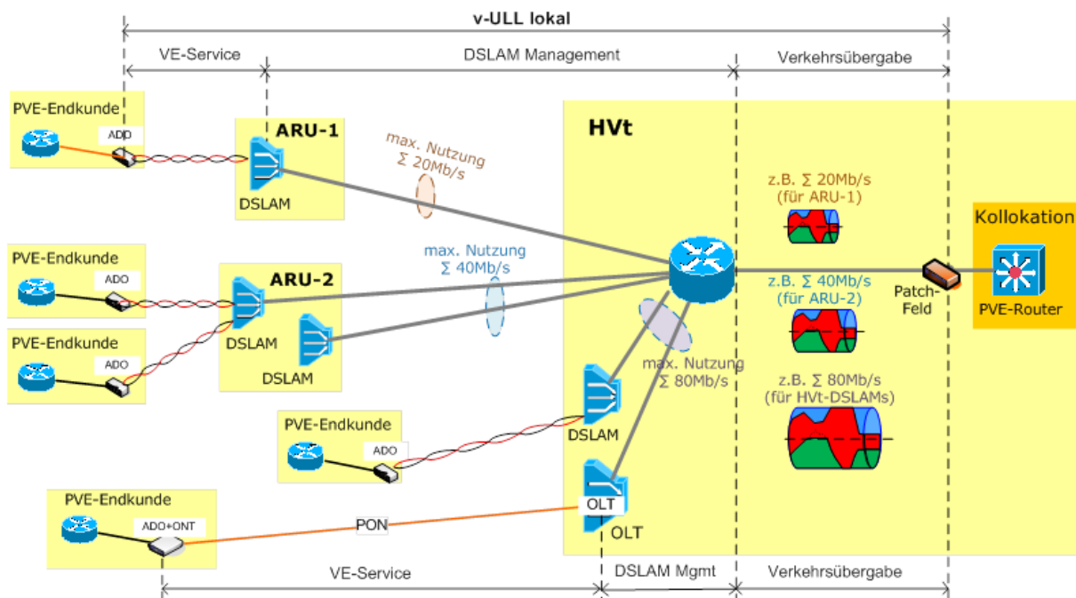
Abbildung 13: DSLAM Management lokal mit (z.B.) 3 möglichen Standorten in einem HVt-Bereich
