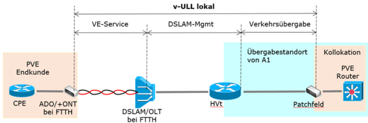
Abbildung 1: v-ULL 2.0 lokal
