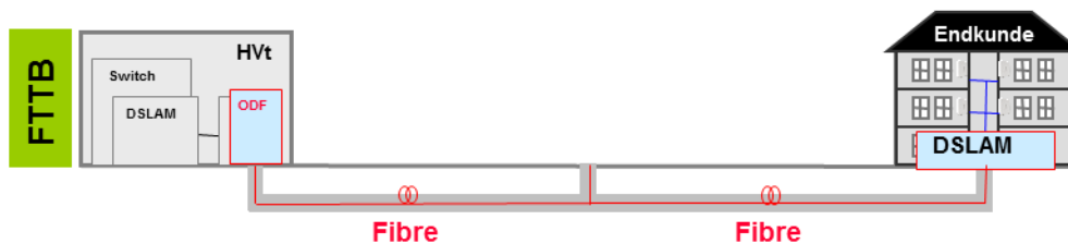
Abbildung 6: FTTB Allgemein
