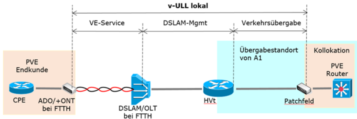
Abbildung 1: v-ULL 2.0 lokal
