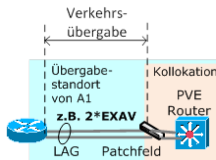
Abbildung 4: Verkehrsübergabe am HVt/Übergabestandort mit 2* EXAV (LAG - geschützte Anbindung)
