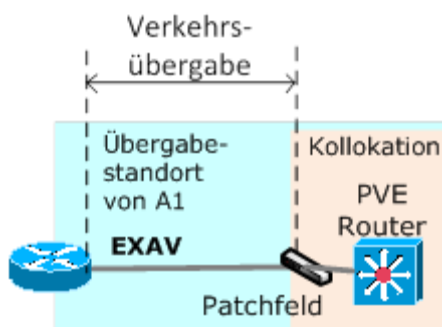
Abbildung 3: Verkehrsübergabe am HVt/Übergabestandort mit EXAV
