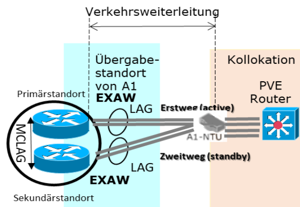
Abbildung 9: Verkehrsweiterleitung zum PVE-Standort mit redundanter Anbindung (MC-LAG) auf einen PVE Router
