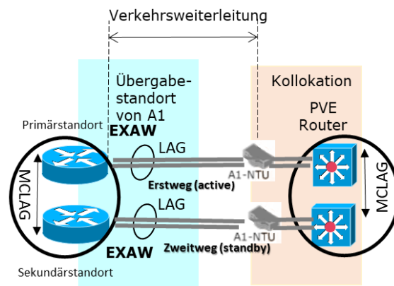
Abbildung 10: Verkehrsweiterleitung zum PVE-Standort mit redundanter Anbindung (MC-LAG) auf zwei PVE Router
