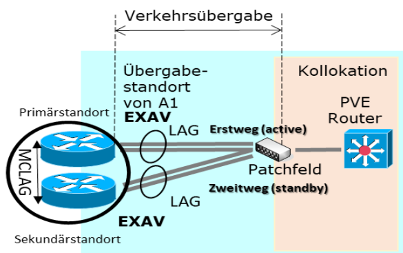
Abbildung 5: Verkehrsübergabe mit redundanter Anbindung am HVt/Übergabestandort mit 2* EXAV (MC-LAG) auf einem PVE-Router
