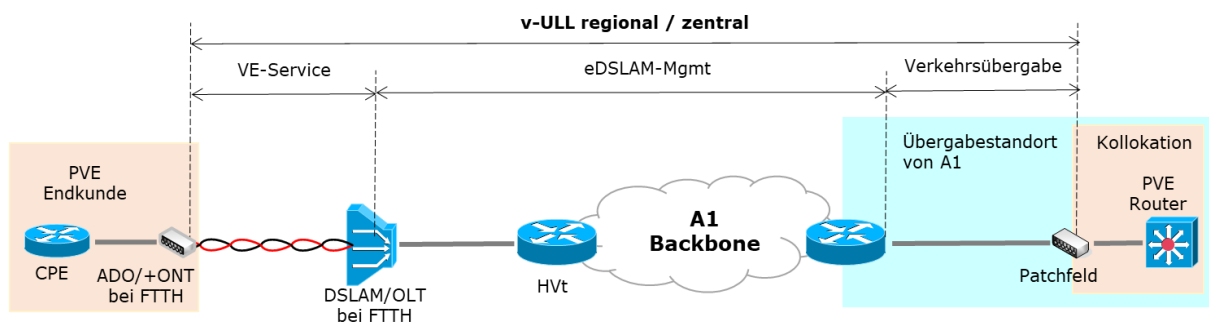
Abbildung 2: v-ULL 2.0 regional
