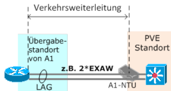
Abbildung 8: Verkehrsweiterleitung zum PVE-Standort mit 2*EXAW (LAG)
