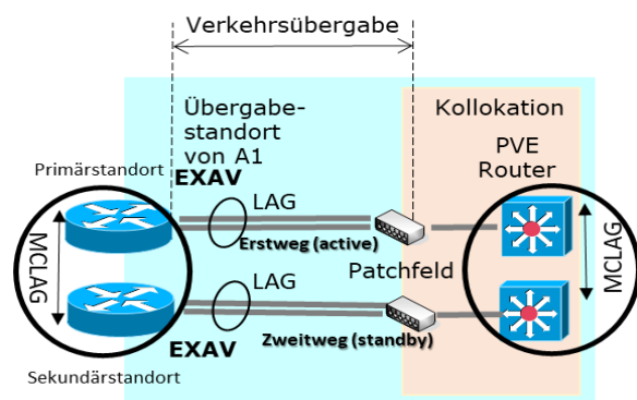
Abbildung 6: Verkehrsübergabe mit redundanter Anbindung am HVt/Übergabestandort mit 2* EXAV (MC-LAG) auf zwei PVE-Routern
