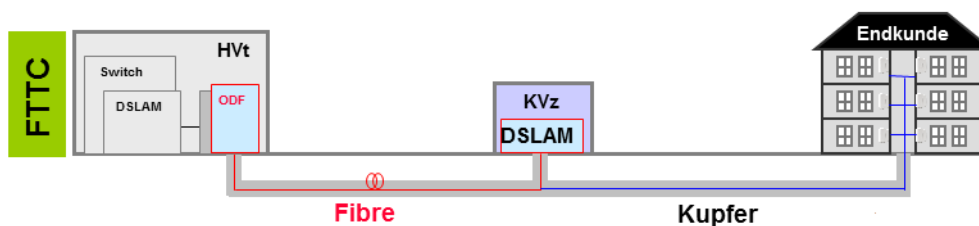
Abbildung 5: FTTC Allgemein
