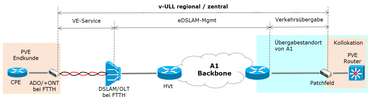
Abbildung 2: v-ULL 2.0 regional sowie zentral
