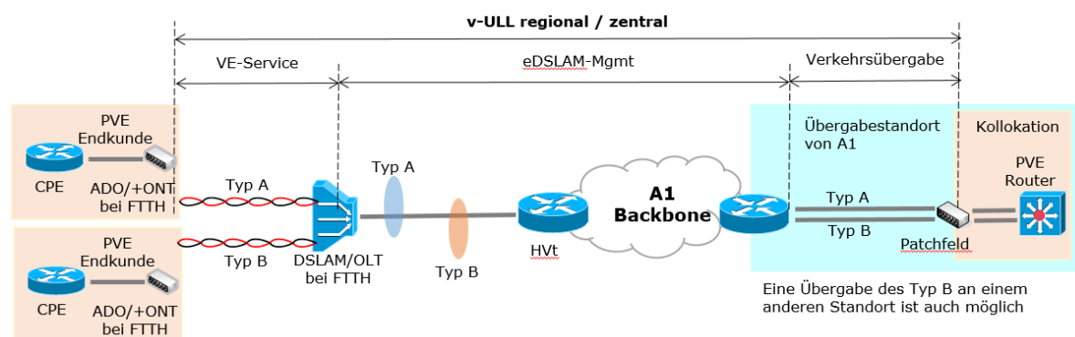
Abbildung 12: enhanced DSLAM Management regional sowie zentral je Standort mit dem A-(e)DSLAM Management und dem B-(e)DSLAM Management mit zwei getrennten Verkehrsübergaben
